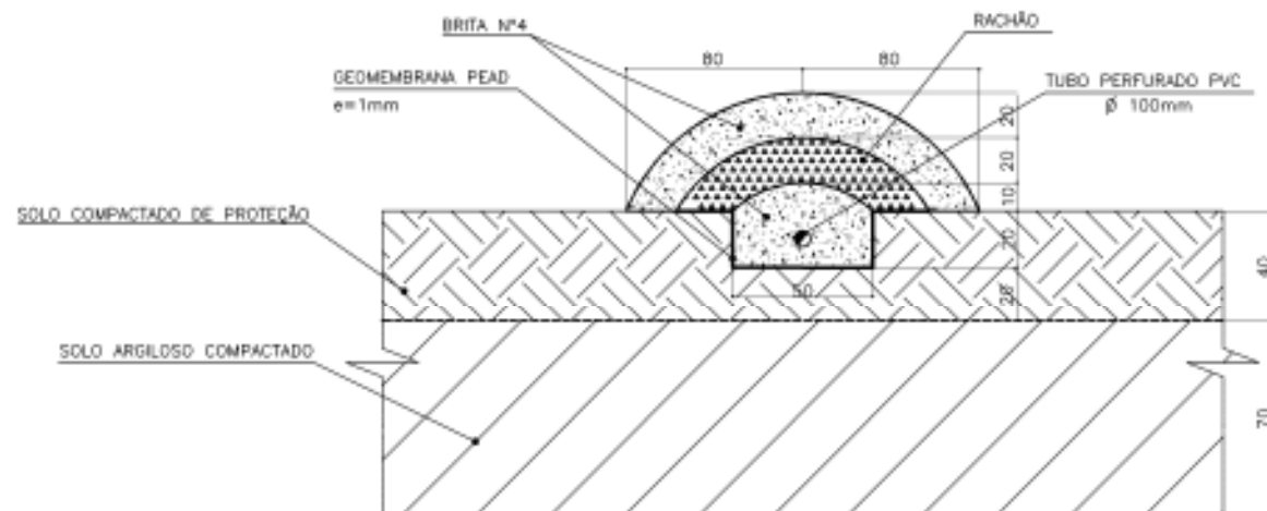
DRENOS DO PERCOLADO - DRENO PRINCIPAL ESCALA = 1:20
