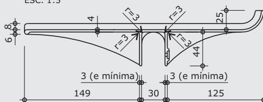
CORTE CC
