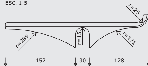
CORTE DD
