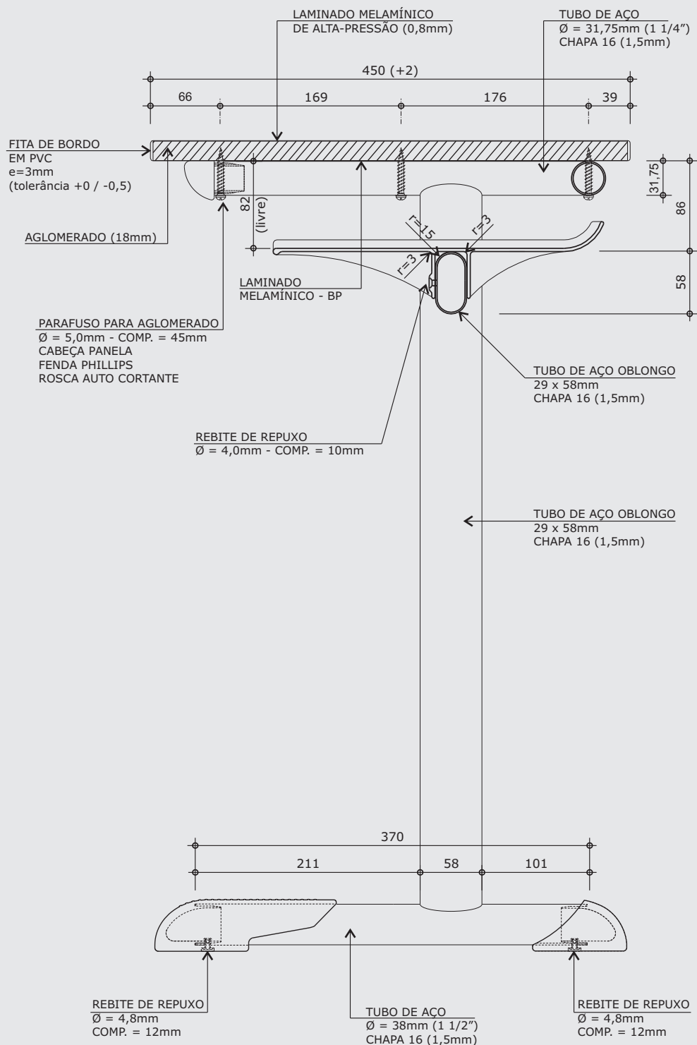
CORTE AA ESC. 1:5
