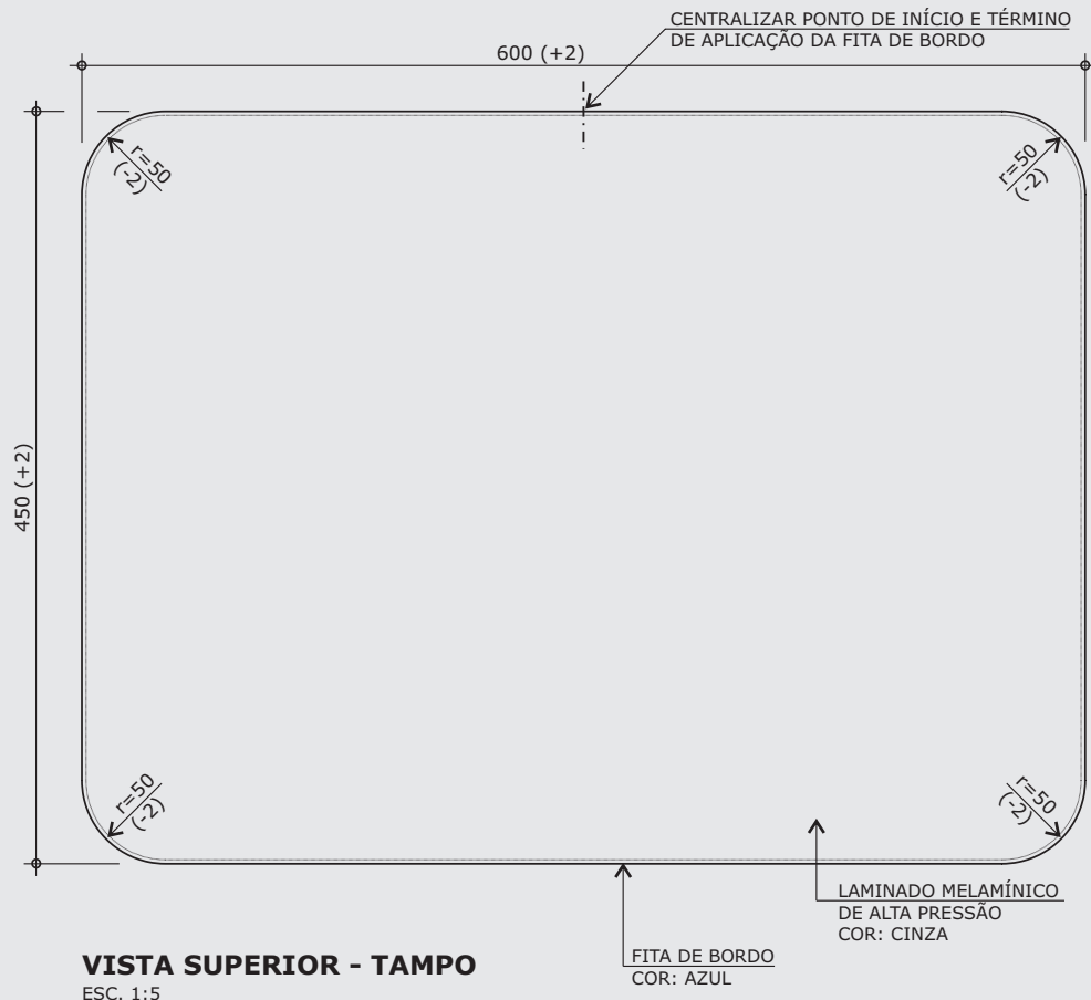
VISTA SUPERIOR
