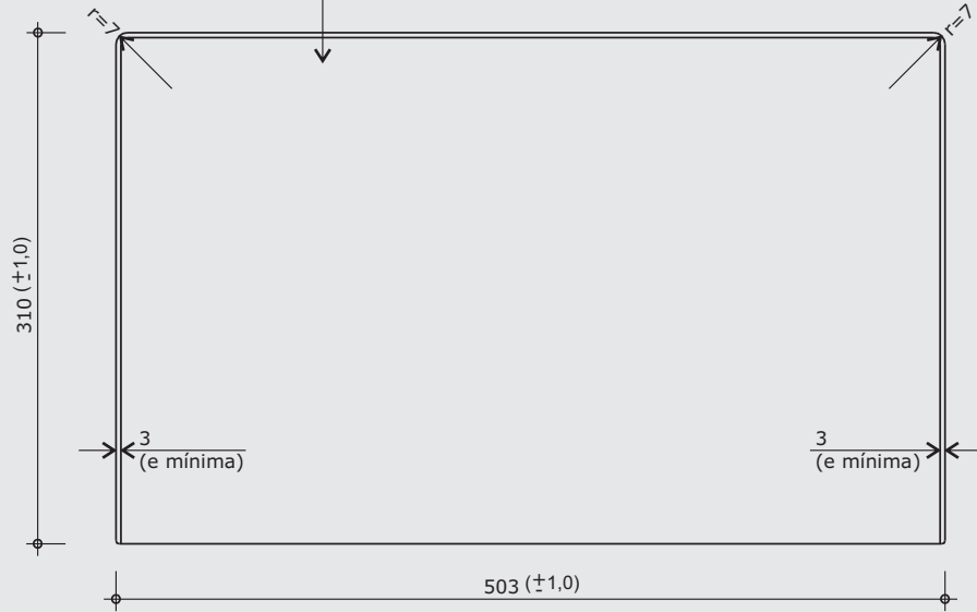
VISTA SUPERIOR
