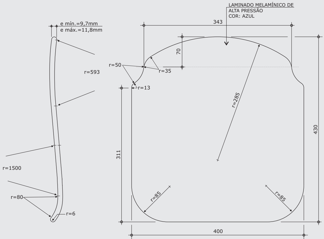
VISTA LATERAL
