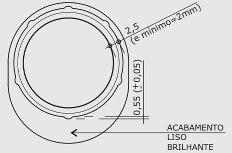
VISTA POSTERIOR ESC. 1:1
