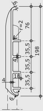
CORTE BB
