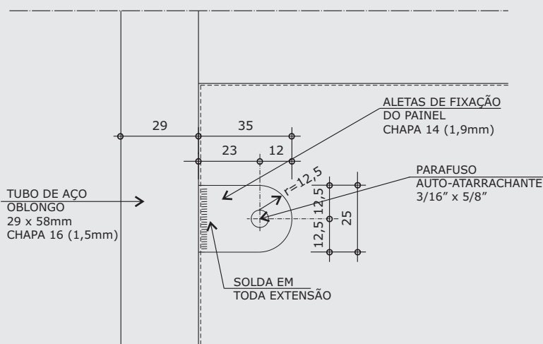
DETALHE 2
