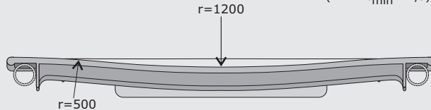
CORTE DD
