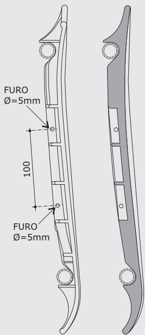
CORTE FF ESC. 1:5
