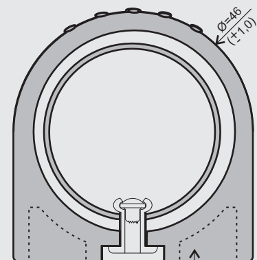
CORTE BB ESC. 1:1 VAZIO NA BASE PARA REDUÇÃO DE MASSA
