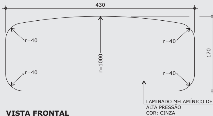
VISTA FRONTAL ESC. 1:5
