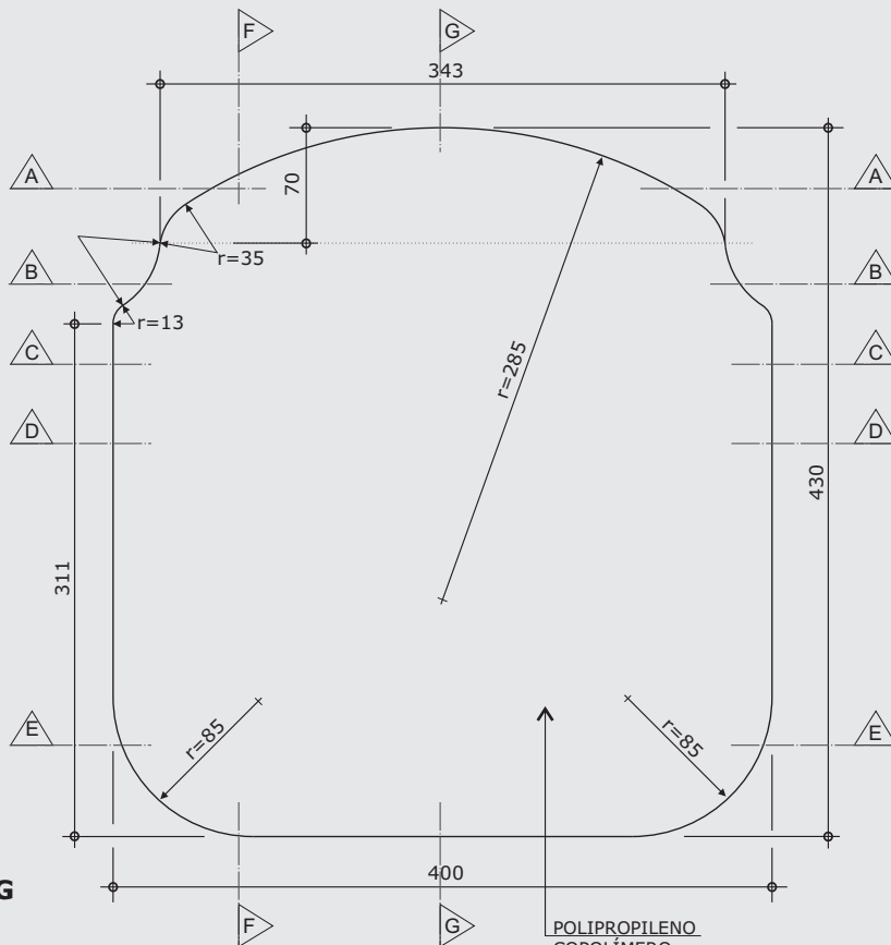
VISTA SUPERIOR
