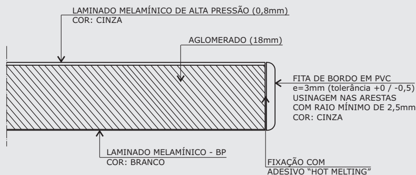
DETALHE 1
