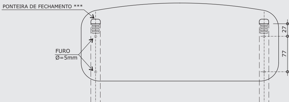
MONTAGEM ESC. 1:5
