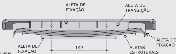
CORTE EE
